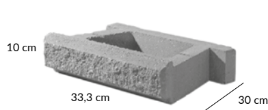
nb | Classic 6° Lite Stone 1/2 WYSOKOŚCI PUSTAKA CLASSIC 6°
