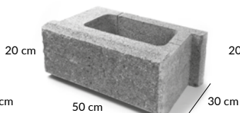
nb | Vertical 3° L 50 BRZEGOWY LEWY 50
