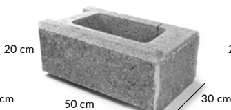
nb | Vertical 3° P 50 BRZEGOWY PRAWY 50
