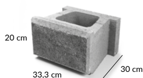
nb | Classic 6° PUSTAK PODSTAWOWY 6°
