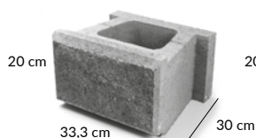
nb | Vertical 3° PUSTAK PODSTAWOWY 3°
