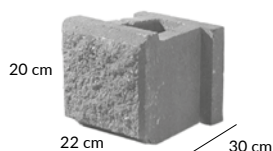
nb | Classic 6° Junior 2/3 DŁUGOŚCI PUSTAKA CLASSIC 6°
